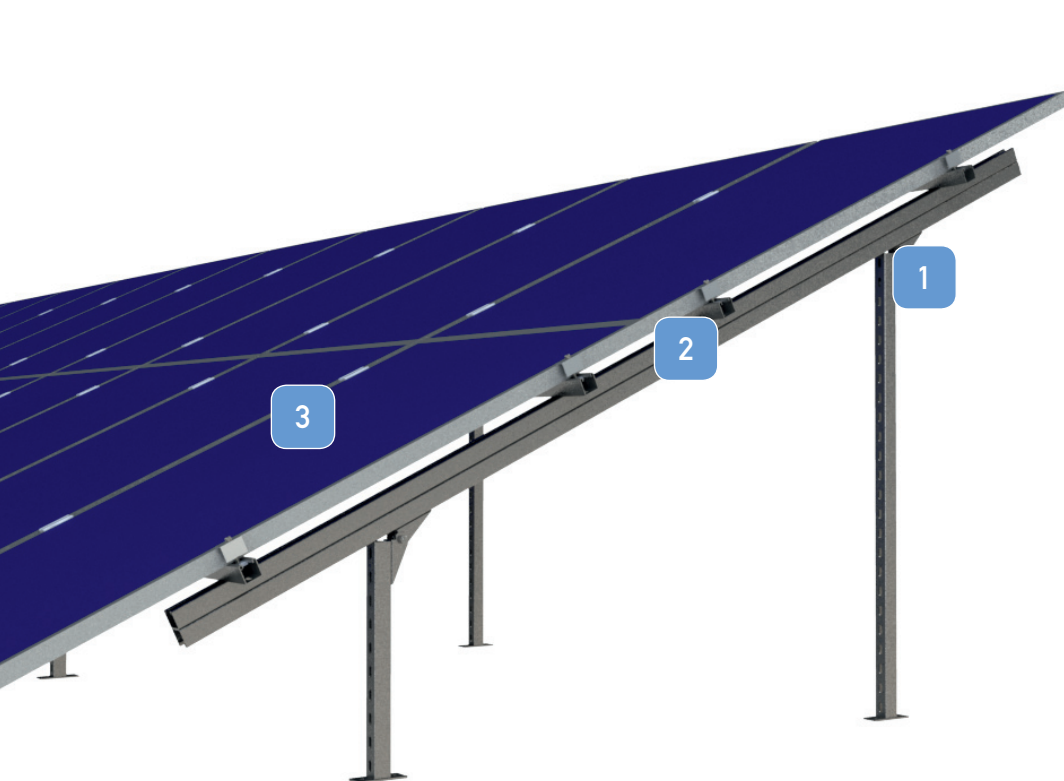
Ejemplo de una estructura en el suelo con materia orgánica elevada a través de la estructura principal
